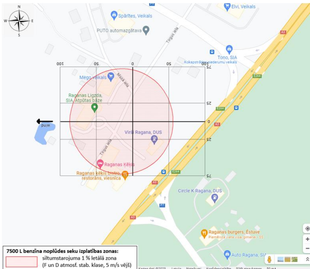
4.5. att. Siltumstarojuma izplatības zona 7500 L noplūduša benzīna gadījumā (ar degšanu)
