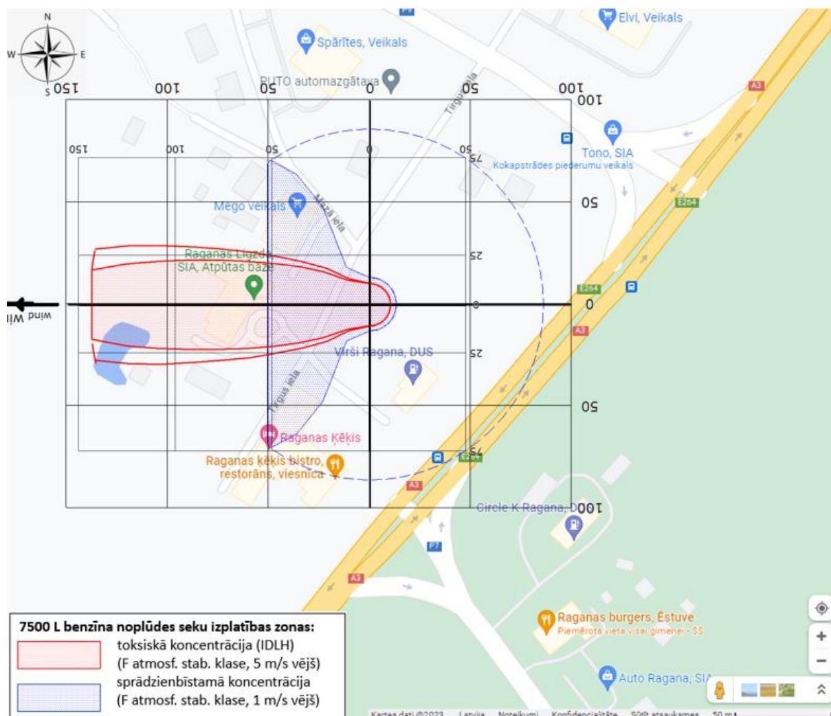
4.4. att. Toksiskās un sprādzienbīstamās koncentrācijas izplatības zonas 7500 L noplūduša benzīna gadījumā (bez degšanas)
