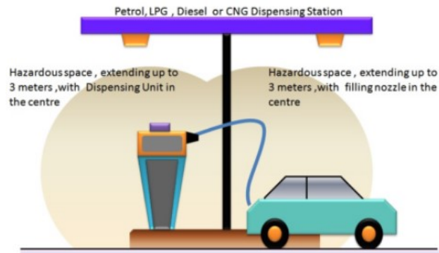
3.3. att. Sprādzienbīstamais zonējums automašīnas uzpildes laikā
