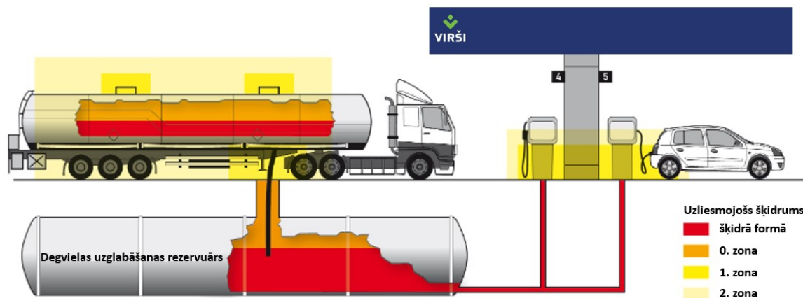
3.1. att. Sprādzienbīstamais zonējums degvielas uzpildes stacijā
