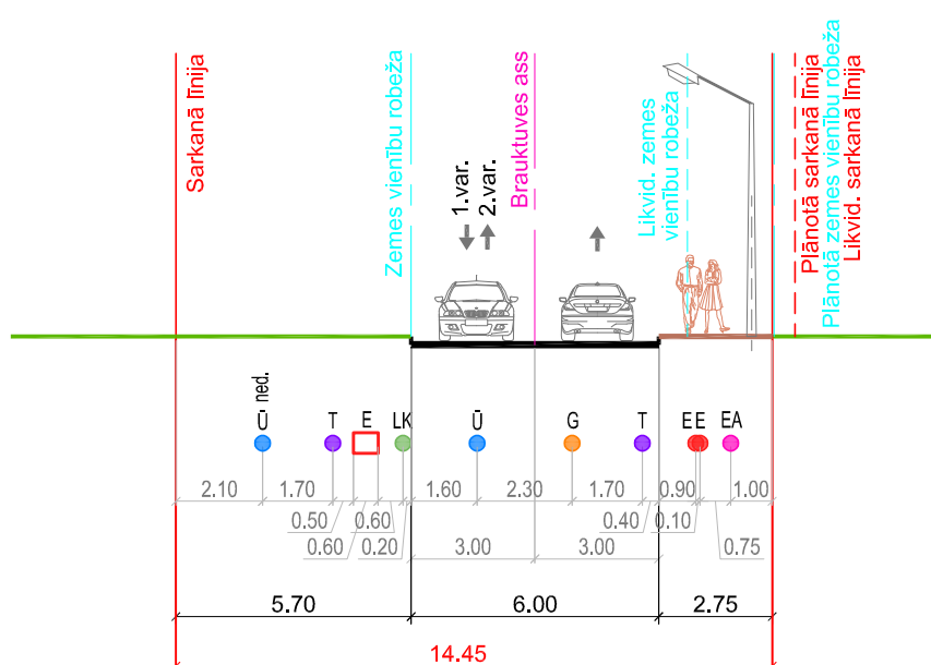
Šķēršprofils 4-4 (Oskara Kalpaka iela)
