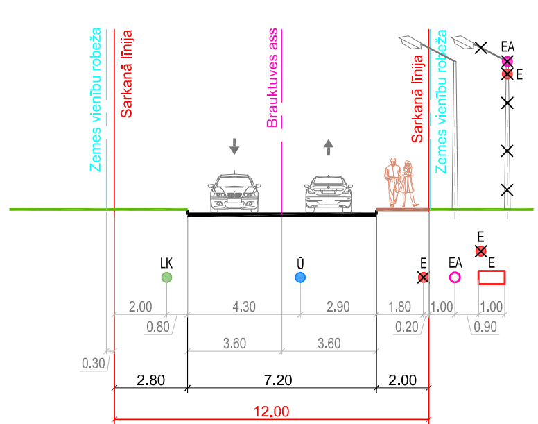
Šķēršprofils 3-3 (Jēkaba Dubura iela)
