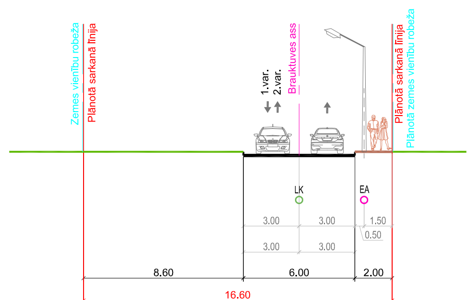
Šķēršprofils 5-5 (Oskara Kalpaka iela)
