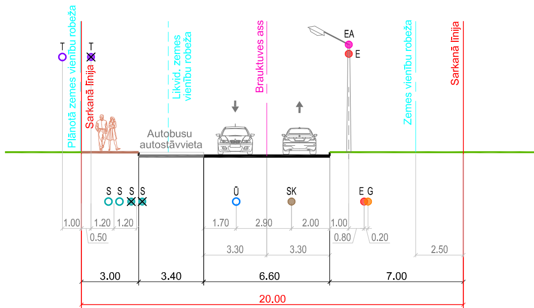
Šķēršprofils 2-2 (Ata Kronvalda iela)
