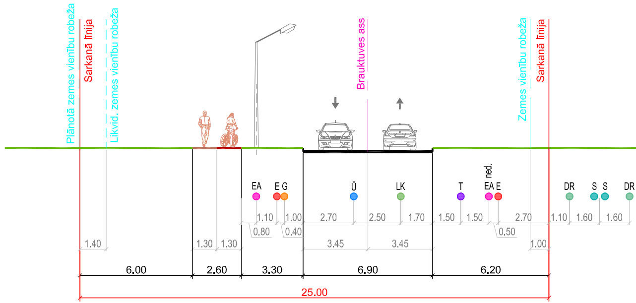
Šķēršprofils 1-1 (Krišjāņa Barona iela)
